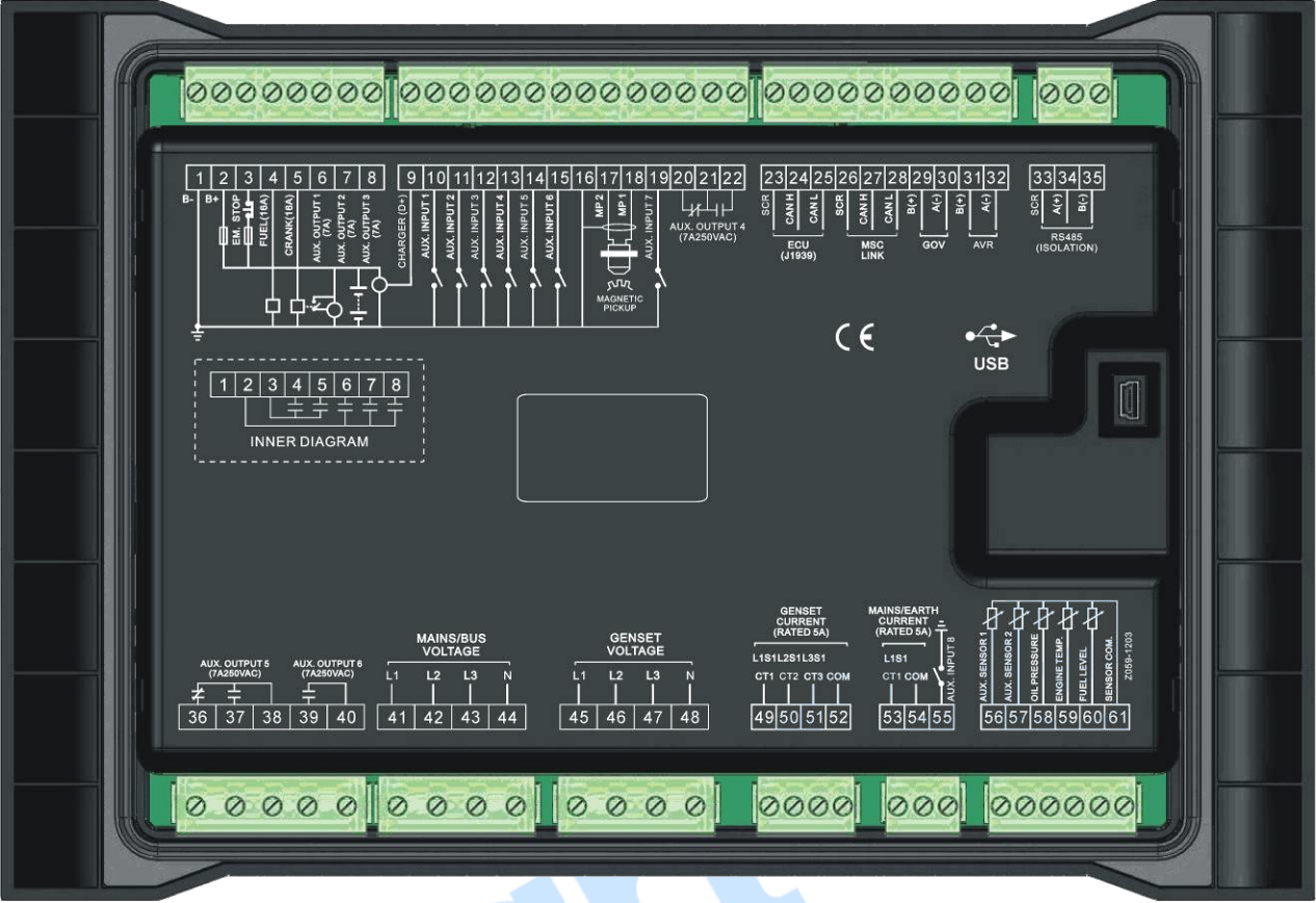
图 2 控制器背面板图
