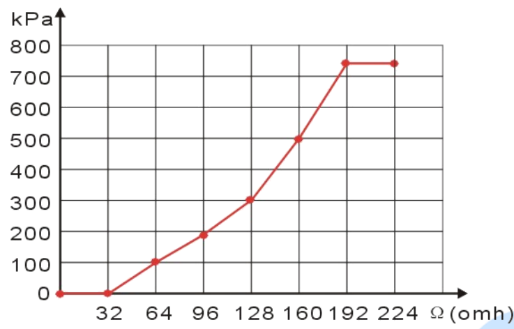
图 3 传感器曲线设置示例图
