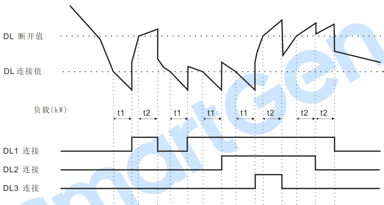
图11 DL 时序
