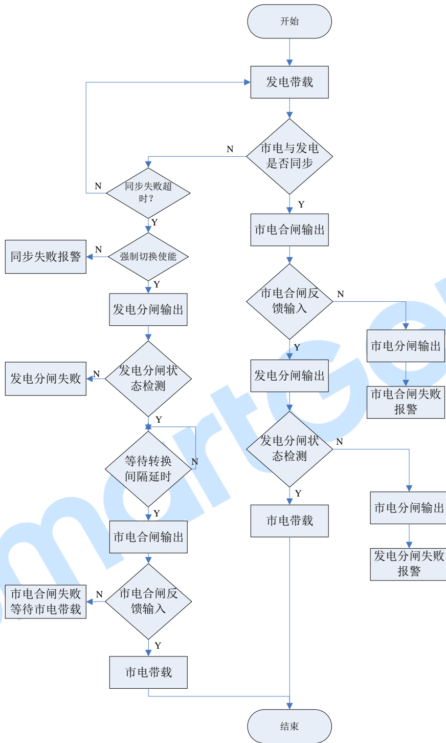
图3 发电带载转市电带载
