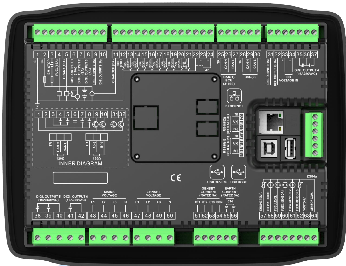
图4 控制器背面板图
