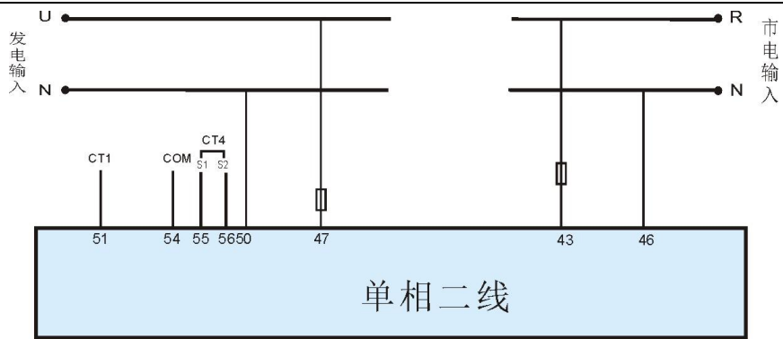
图8 单相二线接线图
