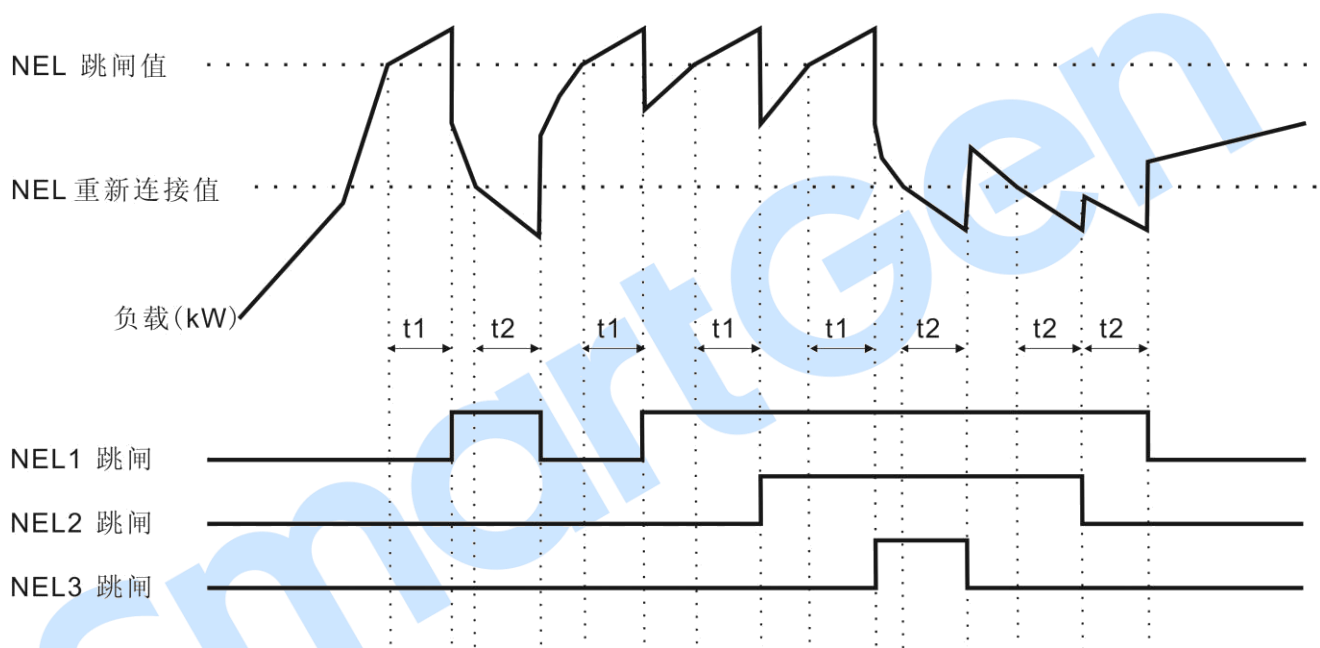
图10 NEL 时序
