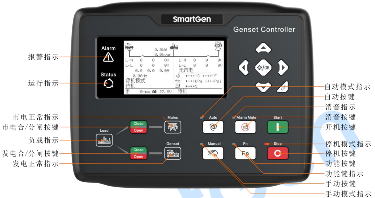
图1 HGM9420N_HGM9420LT 指示灯
