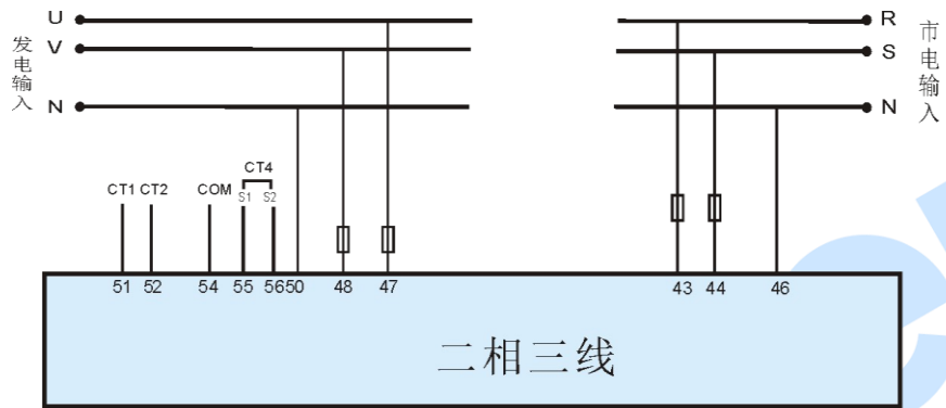
图9 二相三线接线图
