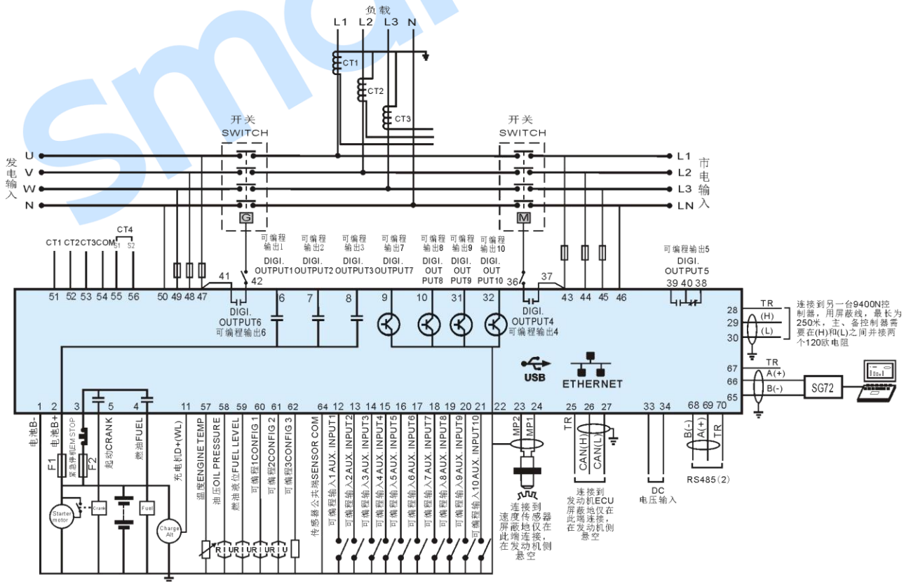
图7 HGM9420N_HGM9420LT 典型应用图
