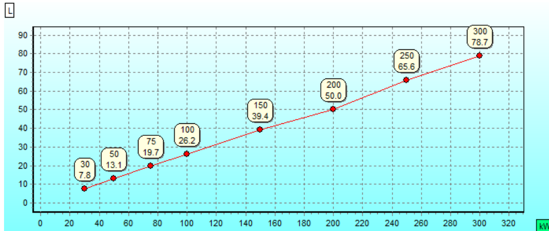
图12 油耗曲线
