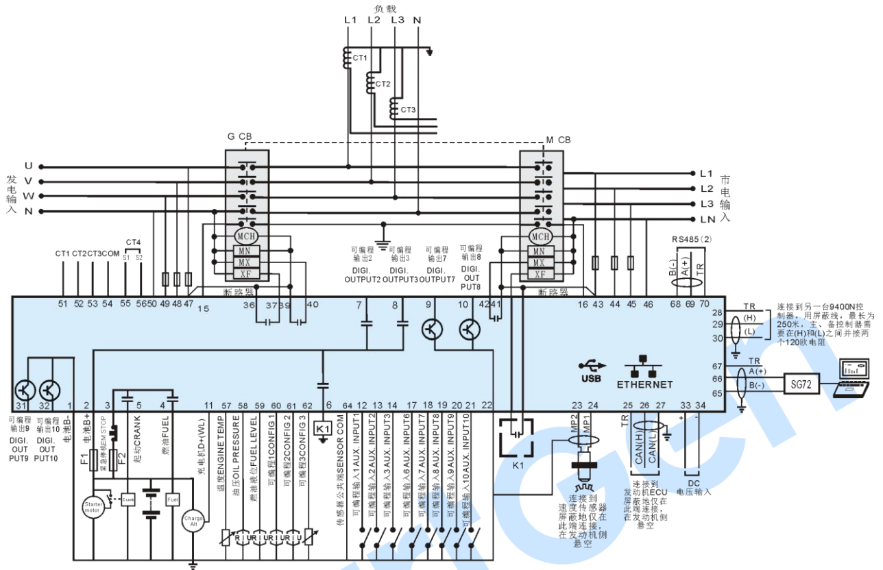
图6 HGM9420N_HGM9420LT 同步切换典型应用图
