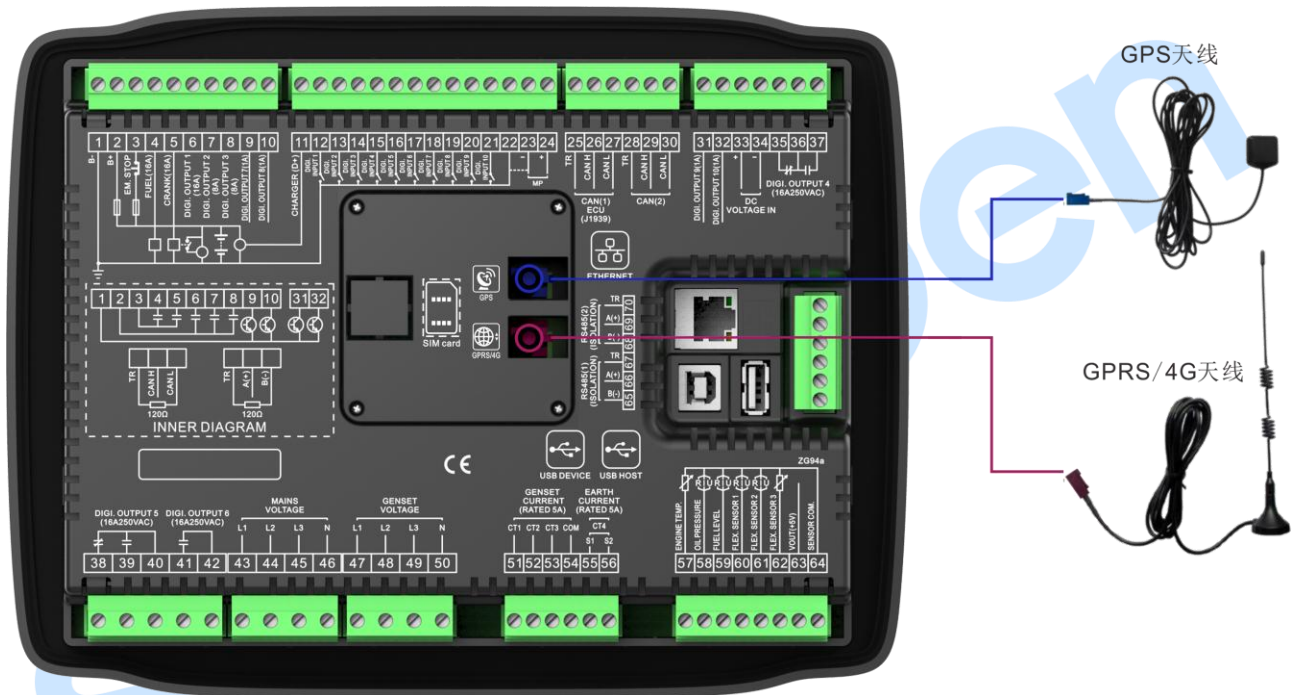
图13 SGE02 天线连接示意图
