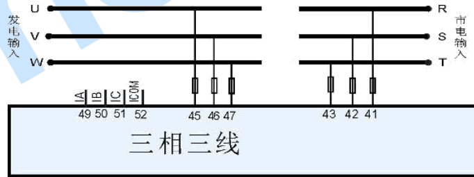
图9 HGM8152 三相三线典型应用图
