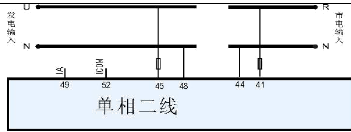
图11 HGM8152 单相二线典型应用图
