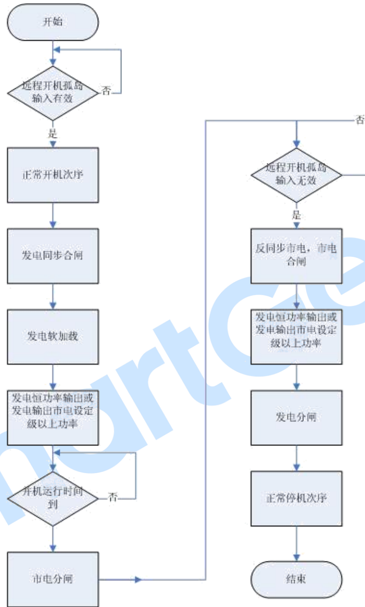
图7 孤岛输出模式
