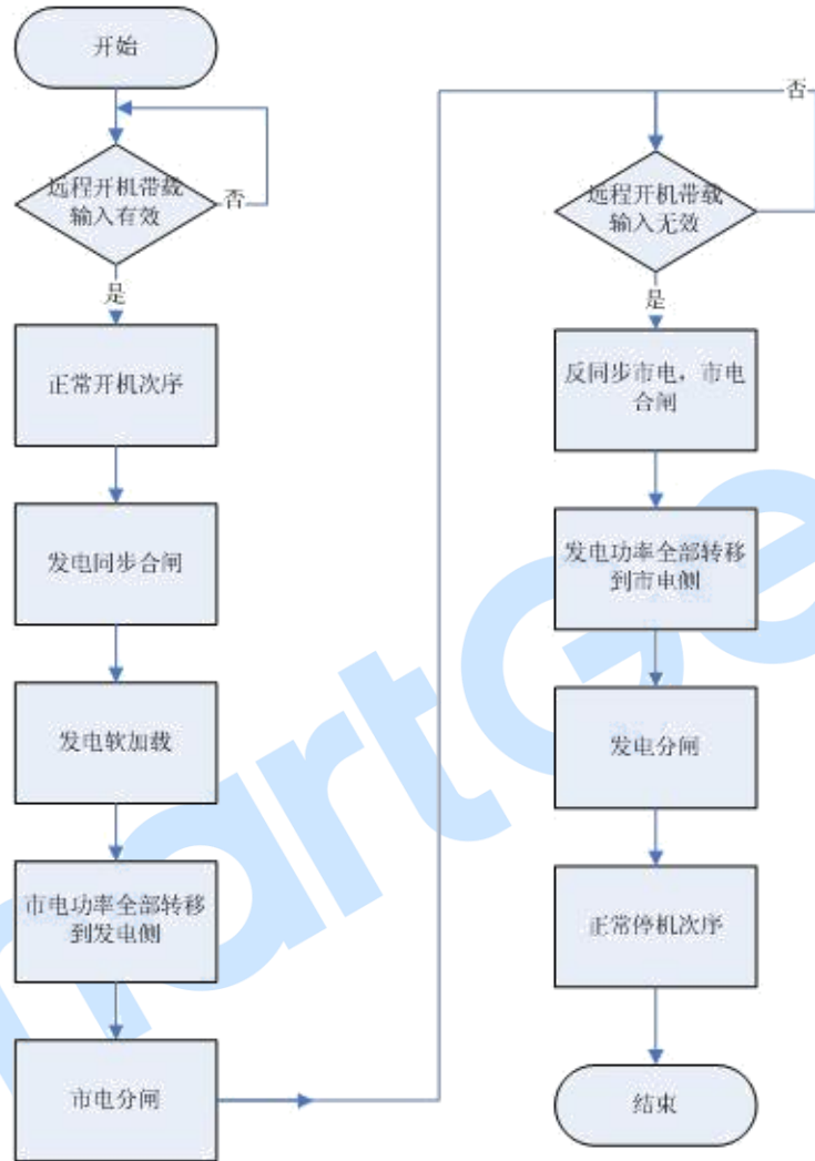
图5 负载接收模式
