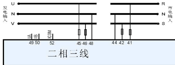
图10 HGM8152 二相三线典型应用图
