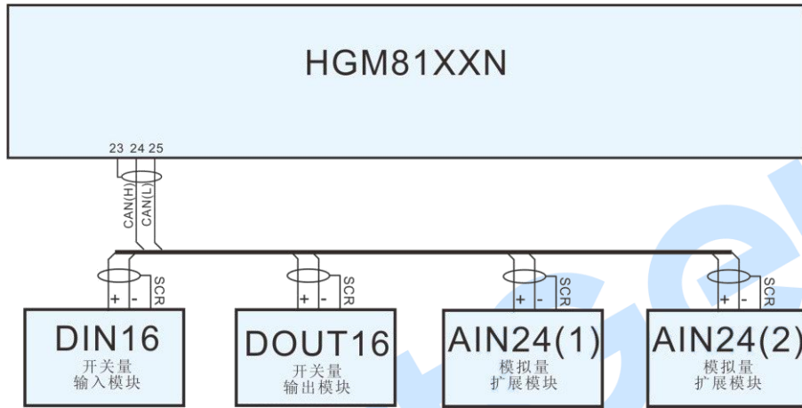
图12 HGM8152 扩展模块典型应用图
