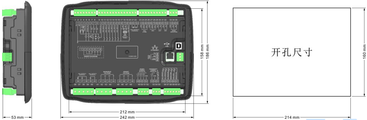
图15 外形及开孔尺寸
