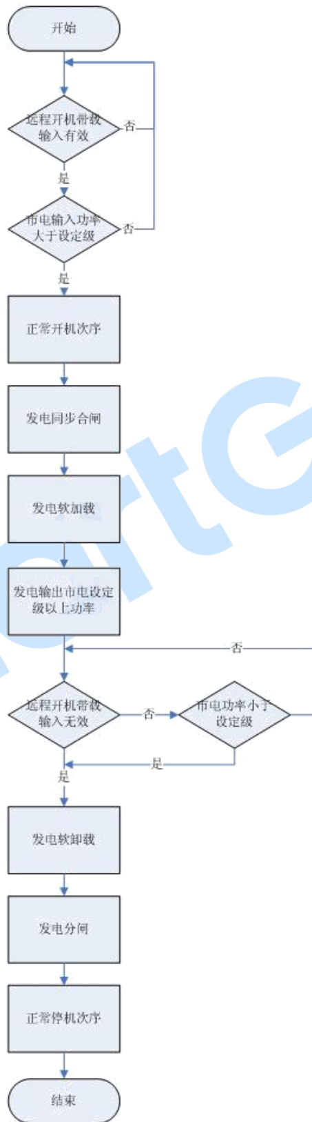
图4 市电剪峰模式
