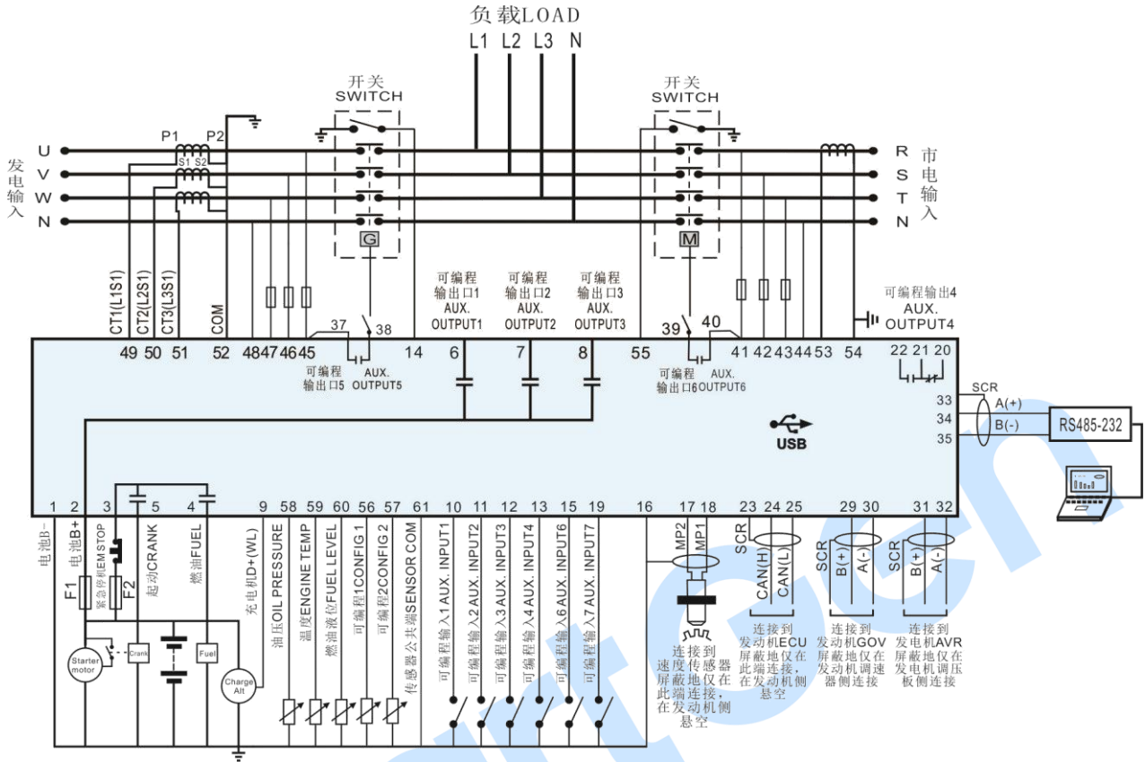
图8 HGM8152 三相四线典型应用图
