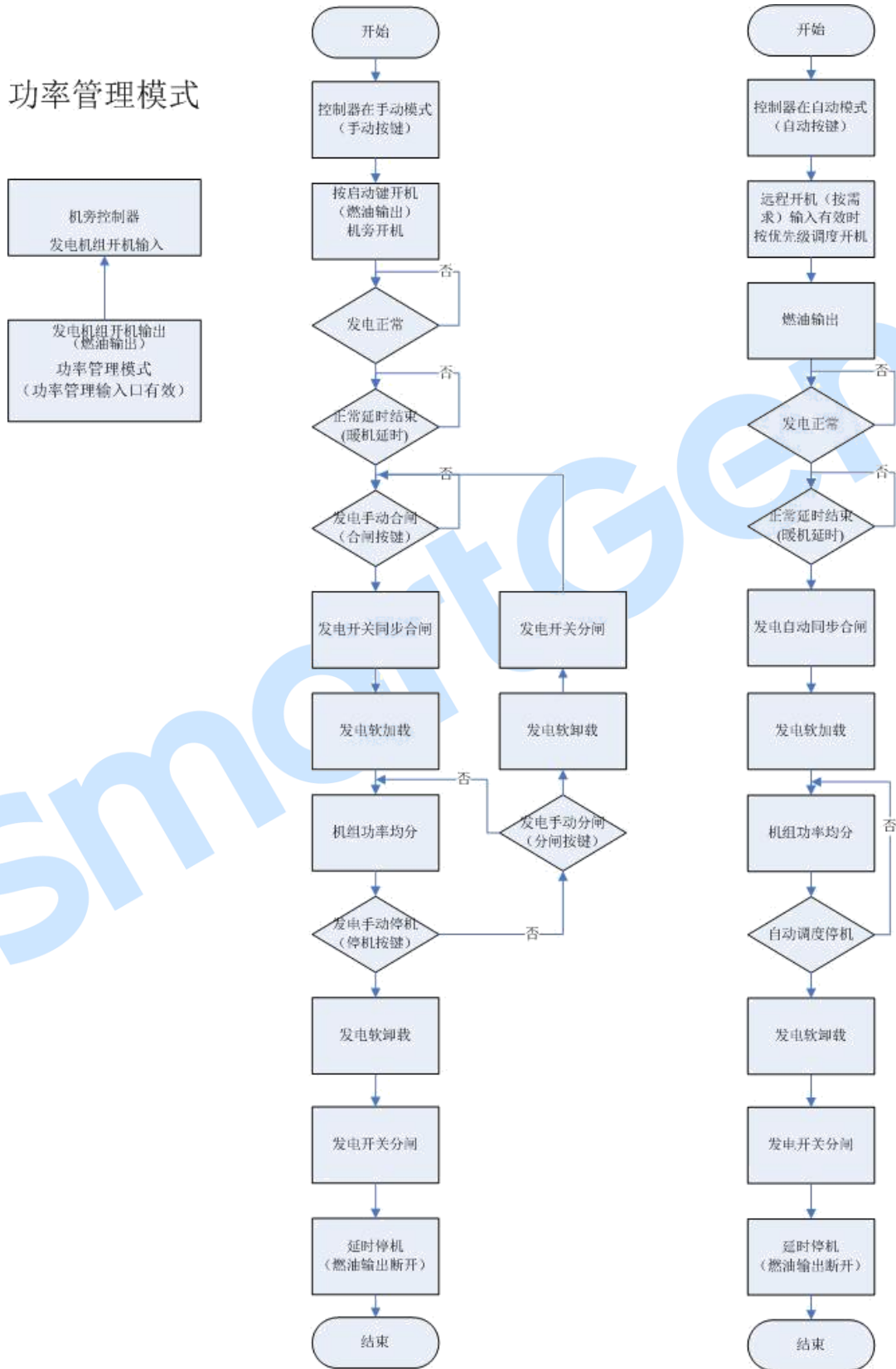
图13 功率管理模式流程图
