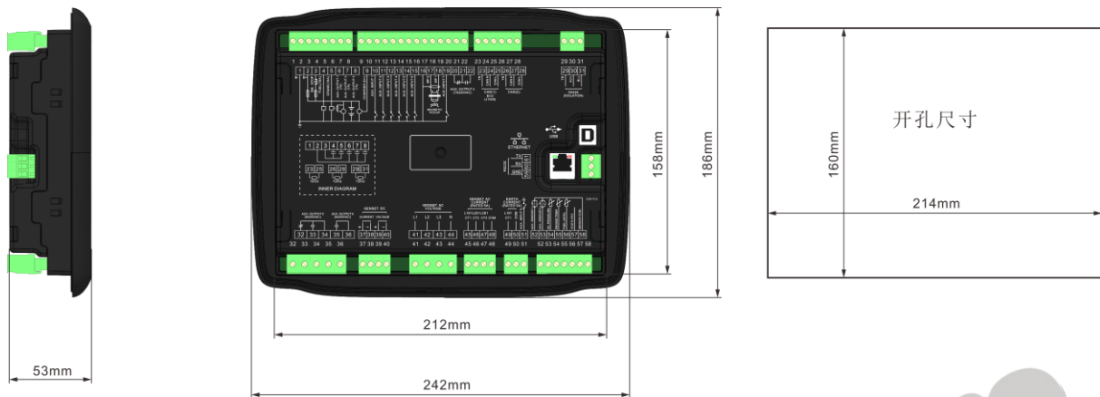
图5 外形及开孔尺寸
