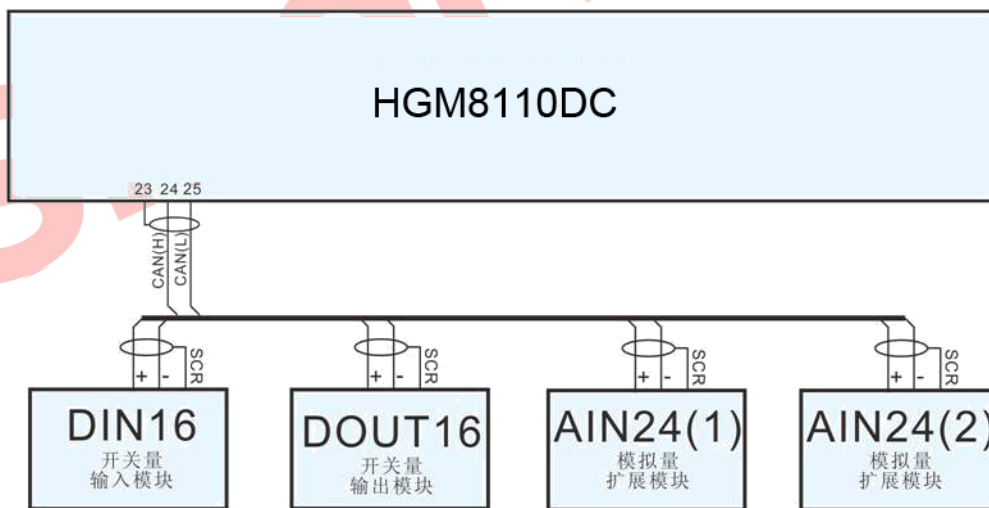
图4 HGM8110DC 扩展模块典型应用图
