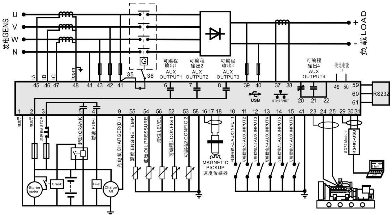
图3 HGM8110DC 典型应用图
