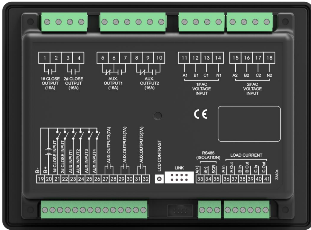
图10 输入输出接口图
