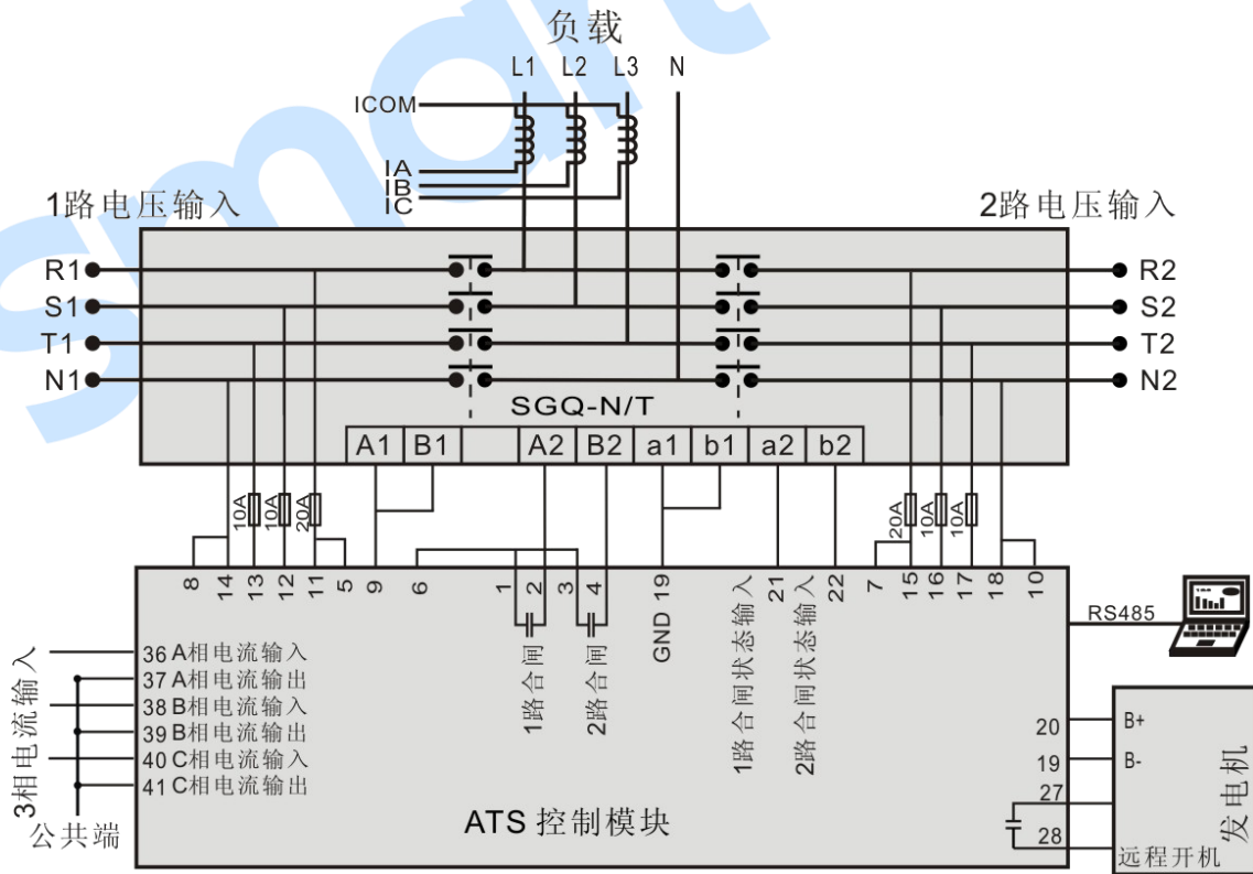
图12 SGQ-N/T 应用图
