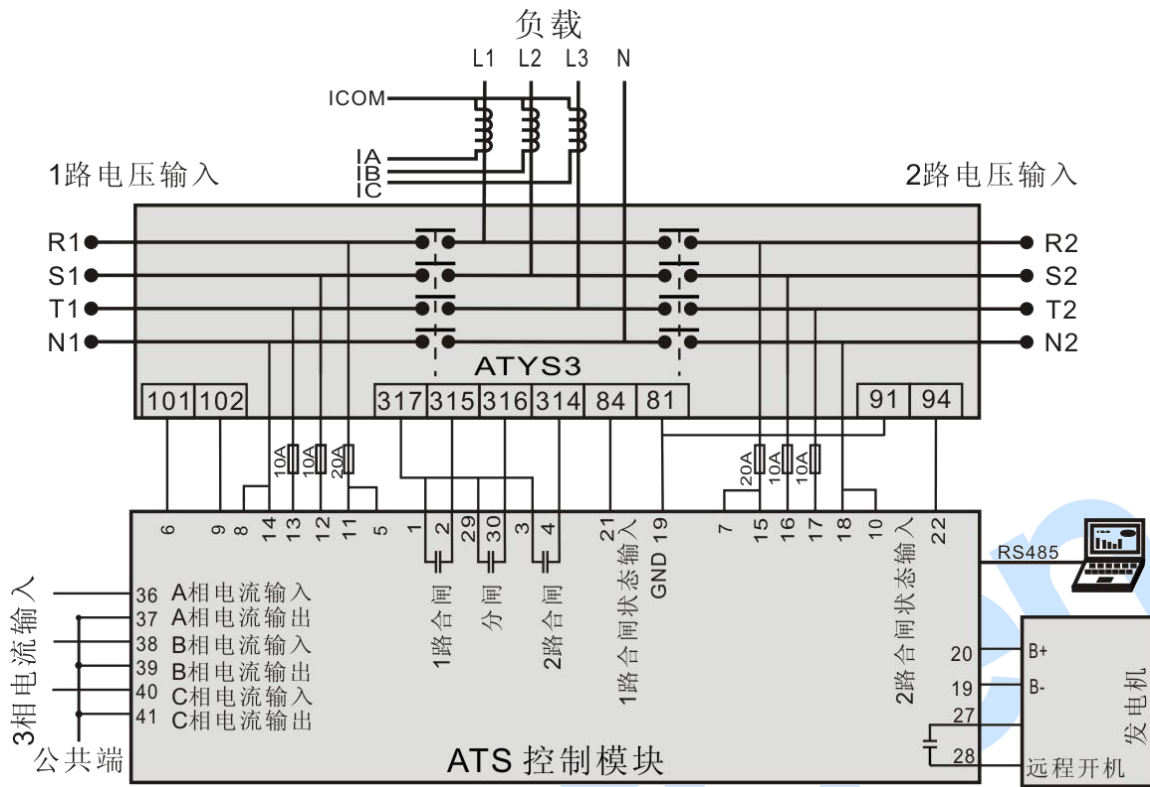
图11 ATYS3 应用图
