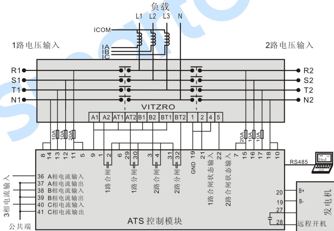
图14 VITZRO 应用图
