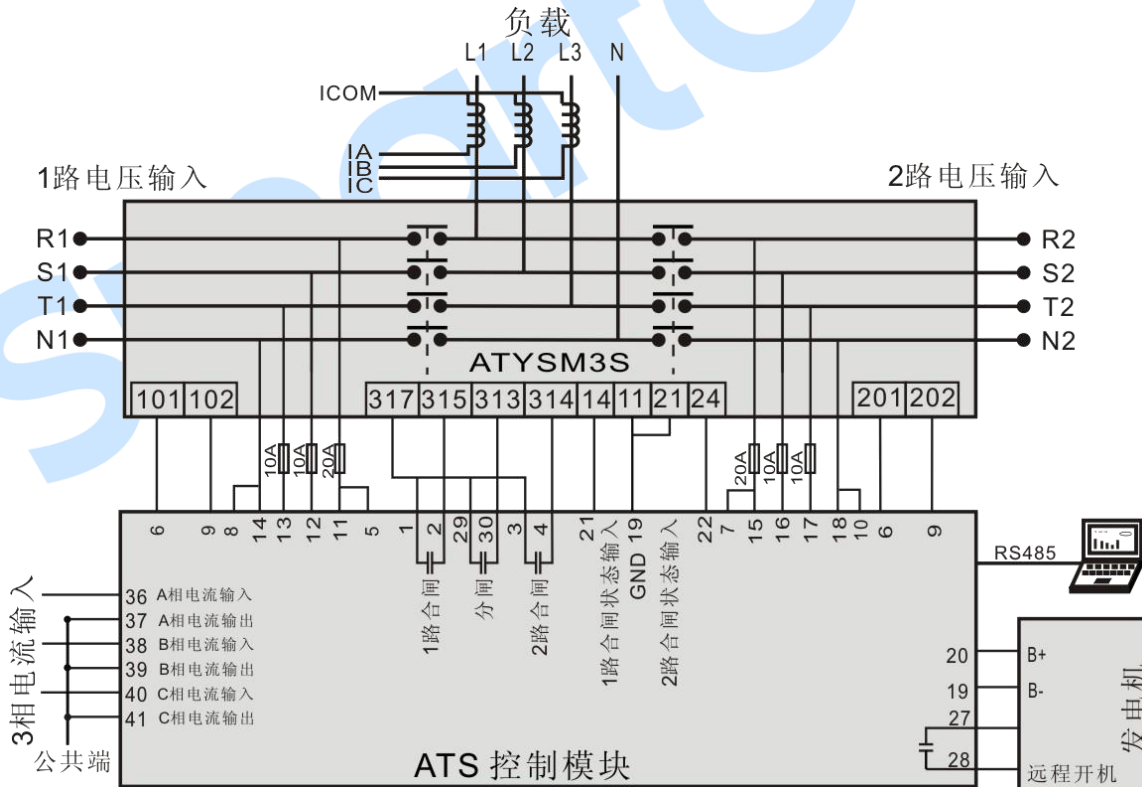
图16 ATYSM3S 应用图
