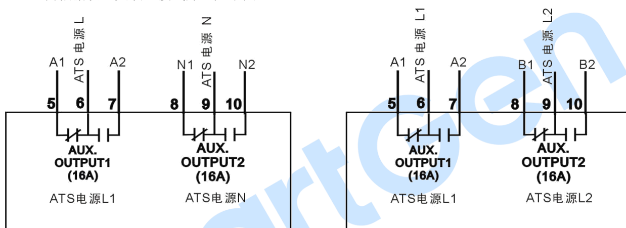
图9 ATS 电源相电压供电和 ATS 电源线电压供电
