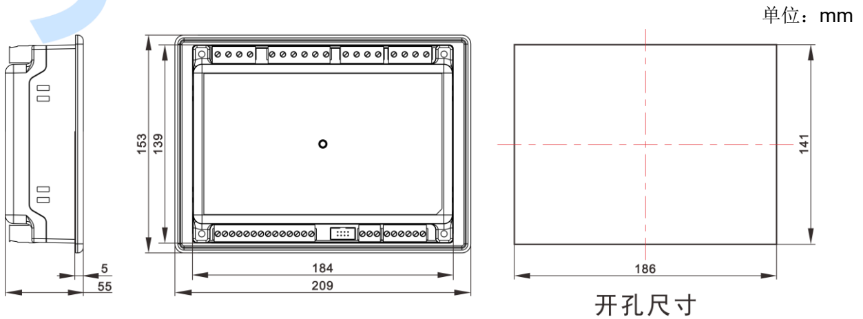
图18 安装尺寸及开孔
