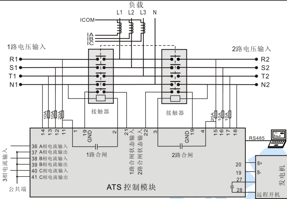
图15 接触器应用图
