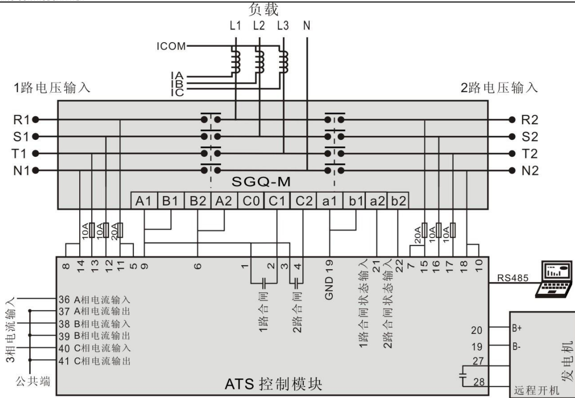
图13 SGQ-M 应用图
