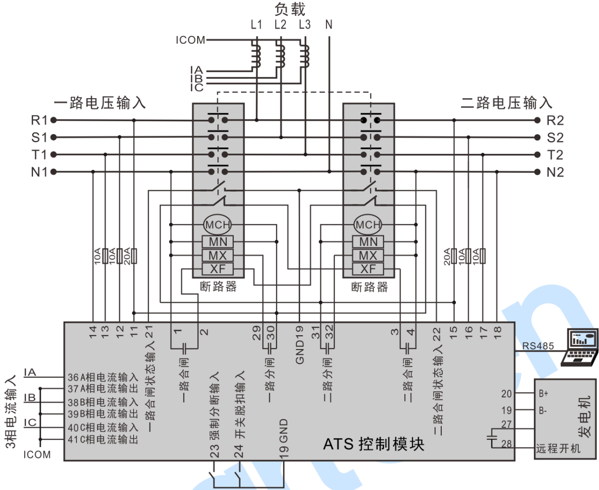
图17 断路器应用图
