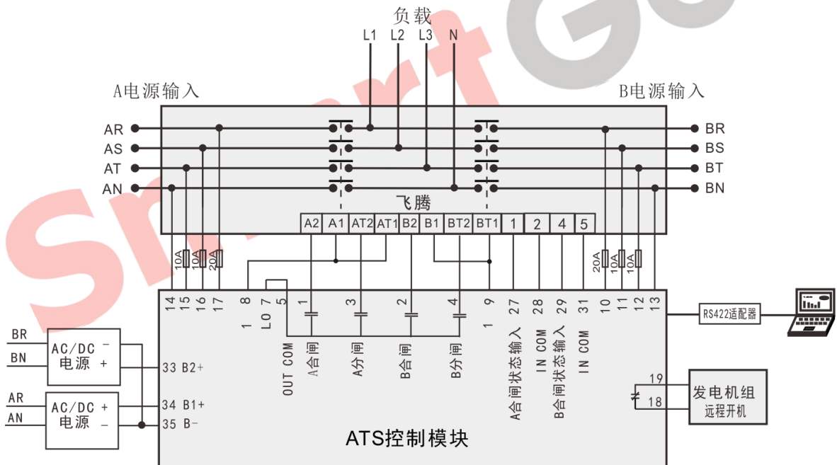
图10 飞腾应用图
