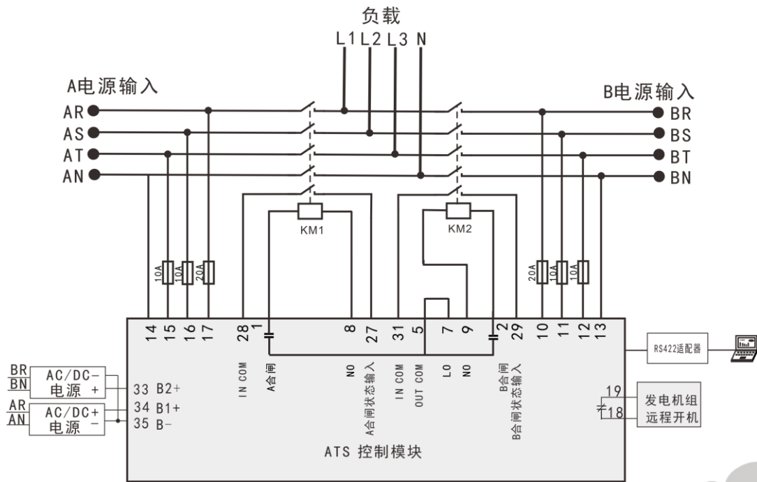
图11 接触器应用图
