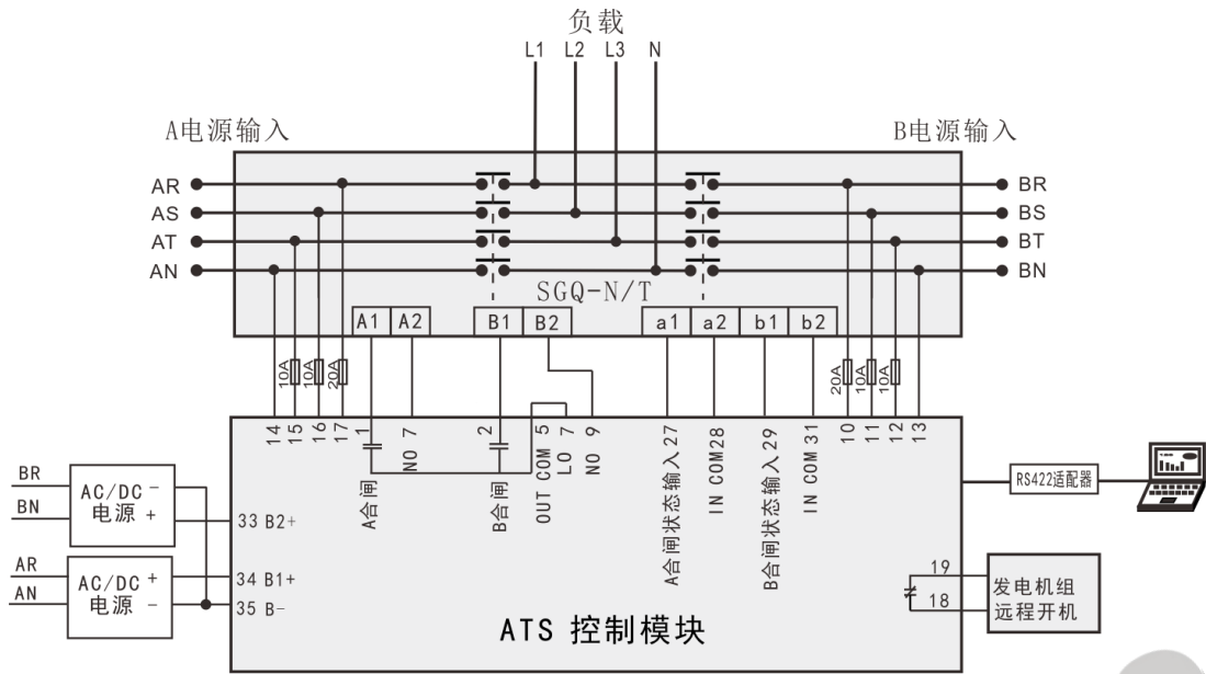
图9 SGQ-N/T 应用图
