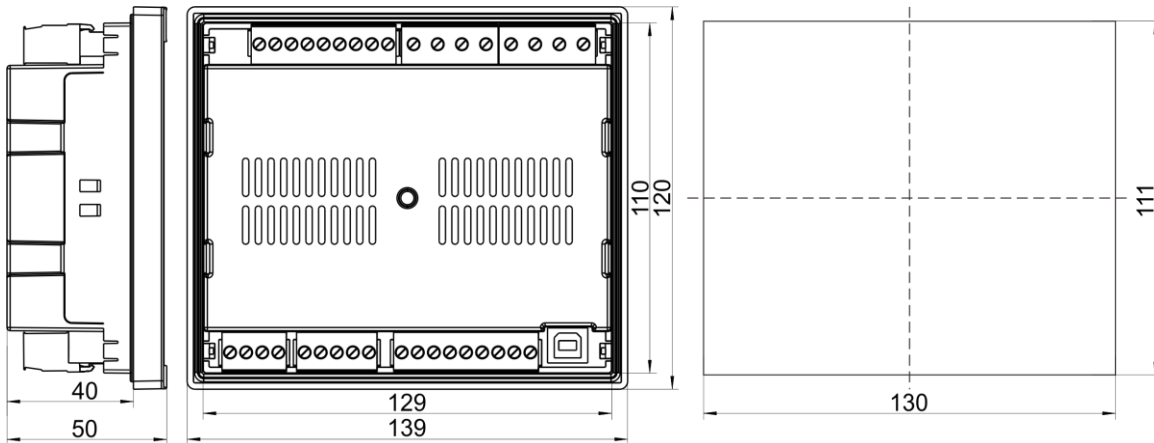
开孔尺寸
