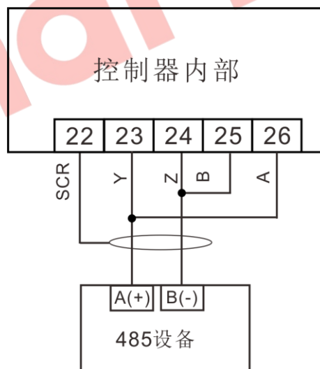
图5 与 485 设备连接示意图
