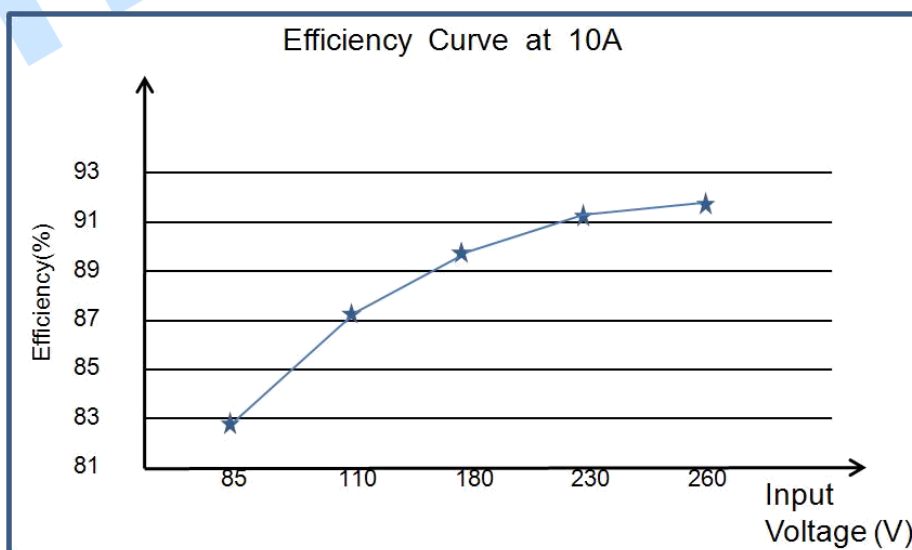
图3 效率曲线
