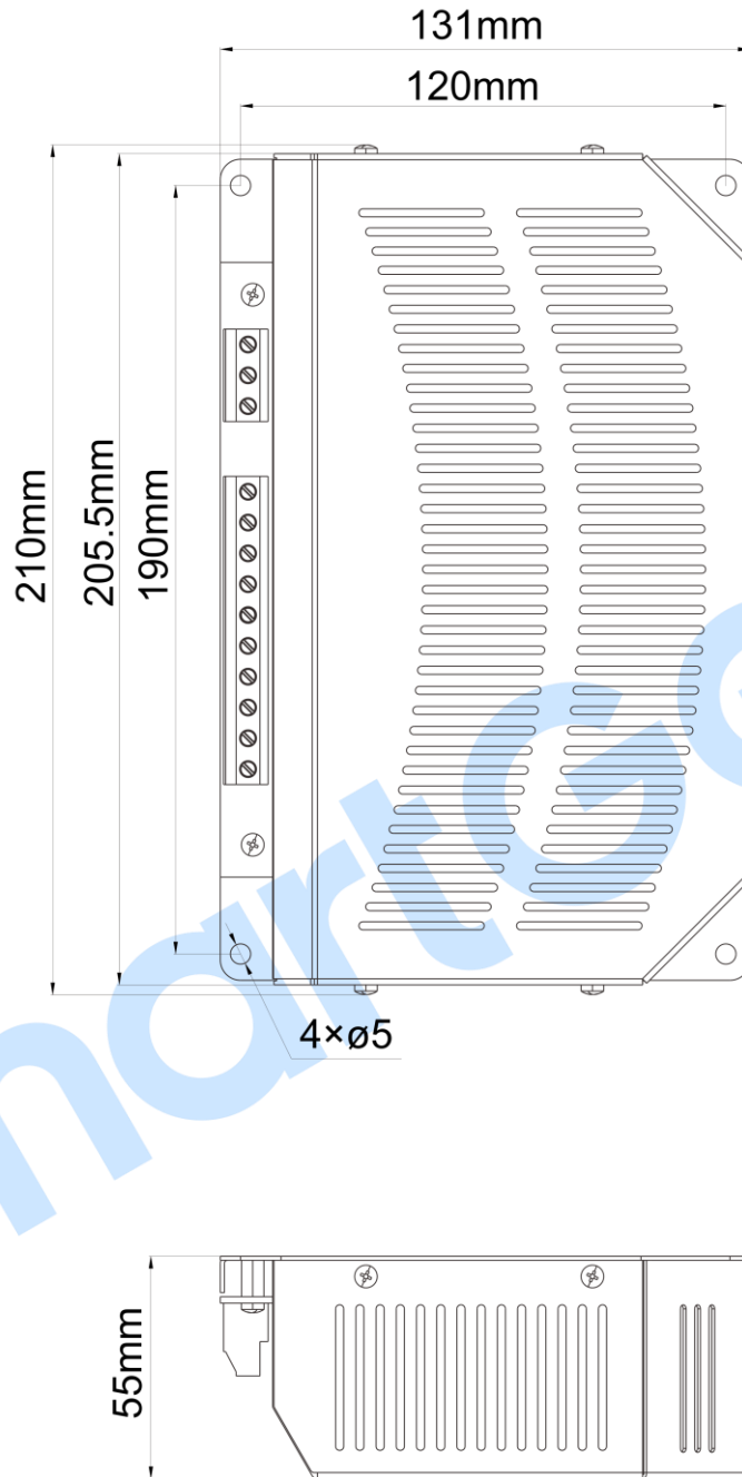
图6 BACM2410 安装尺寸图
