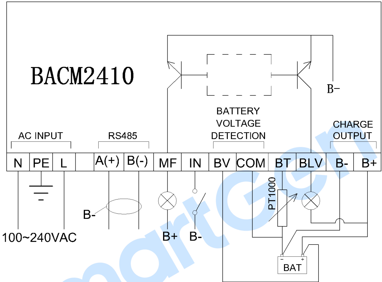
图5 接线图
