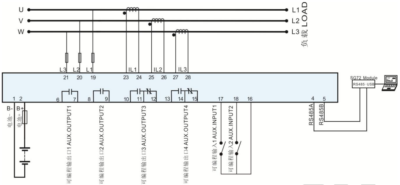
图2 HMP300 典型应用图
