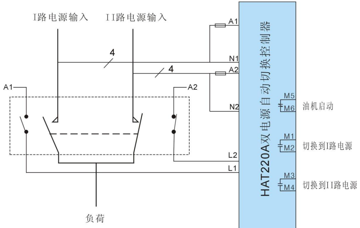
单相二线制应用接线图
