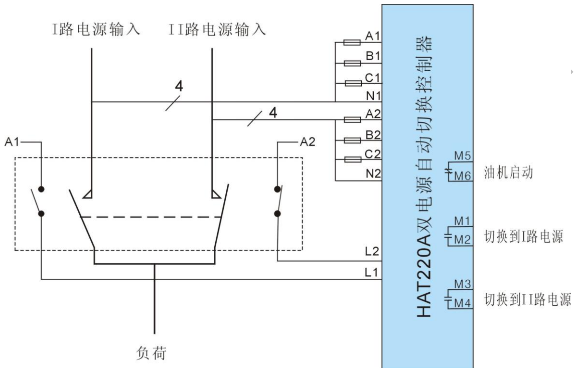
三相四线制应用接线图
