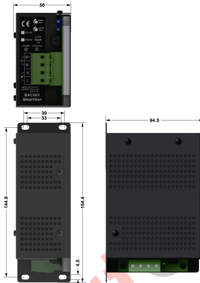
图5 BAC06V 安装尺寸图
