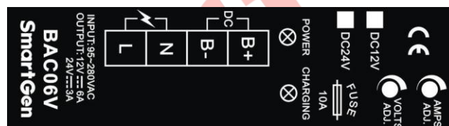
图3 BAC06V 面板图
