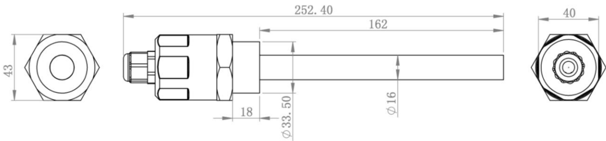
图1 外型及安装尺寸
