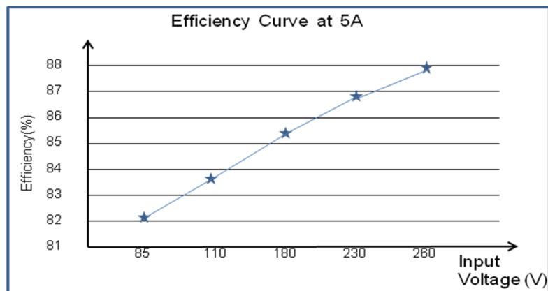
图2 效率曲线
